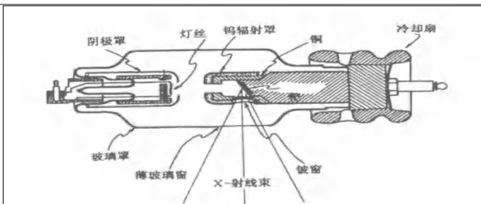
图2-4 典型的X射线管结构图
