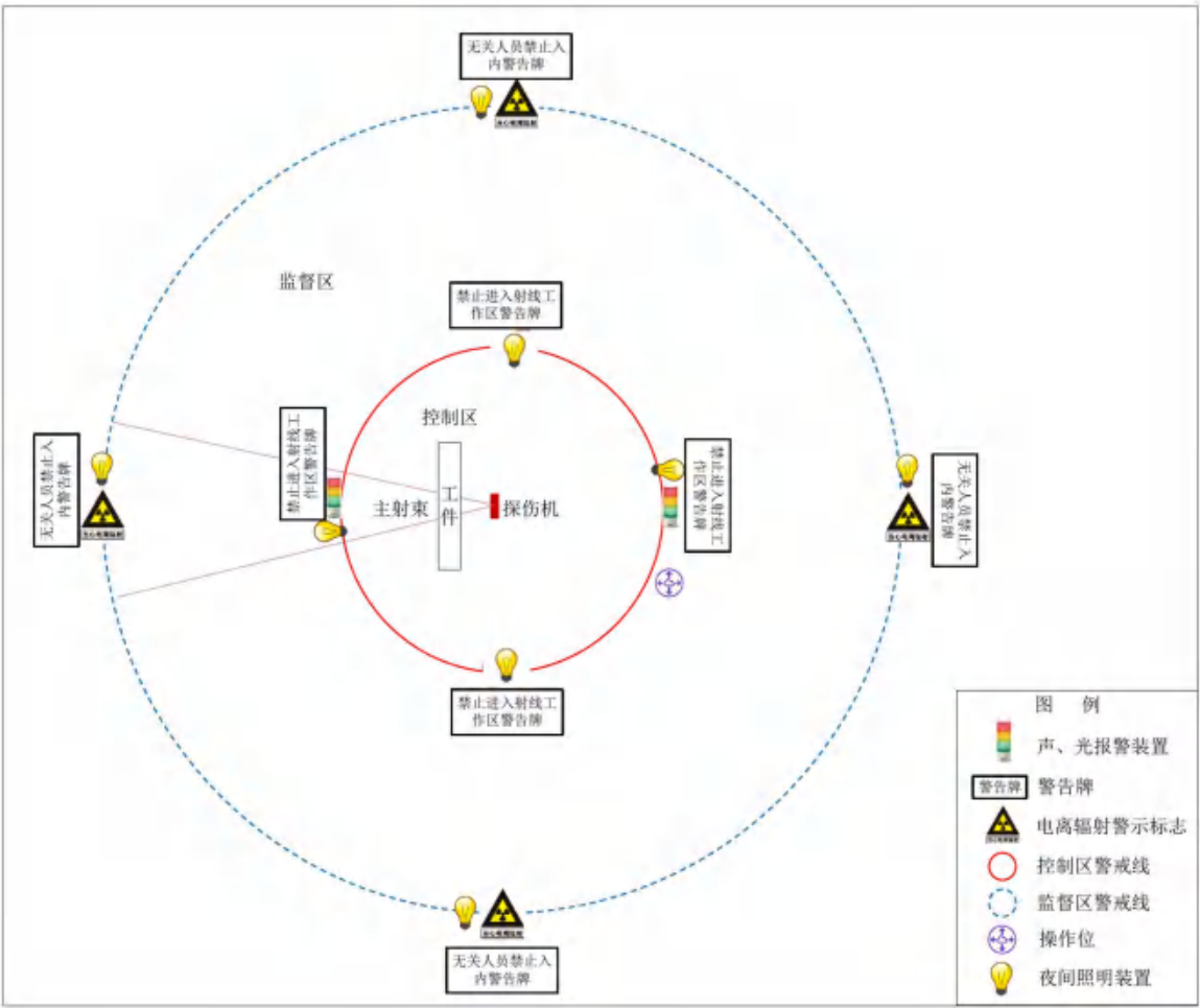
图 3-1 X 射线移动式探伤现场分区及警示标识示意图
