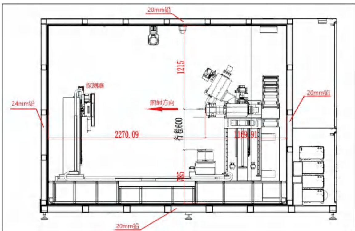
图 3-6 铅房剖面图
