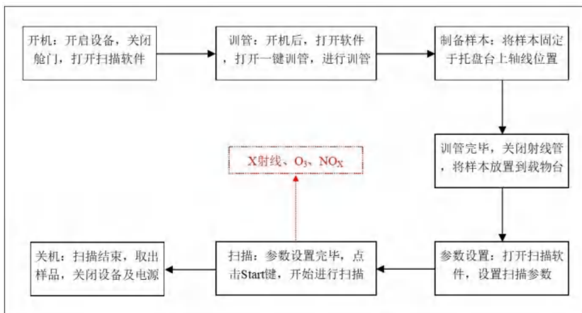
图 3-9 微焦点 X 射线工业 CT 系统工作流程及产污环节图
